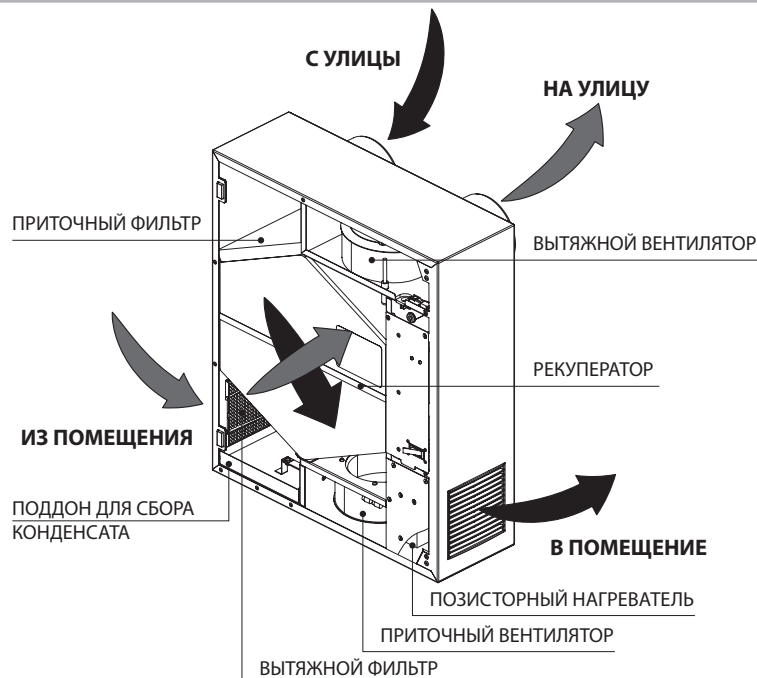
Рис. 2. Компоновка и принцип работы
