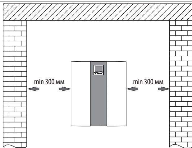
Рис. 3. Минимальные расстояния расположения установки от поверхностей
